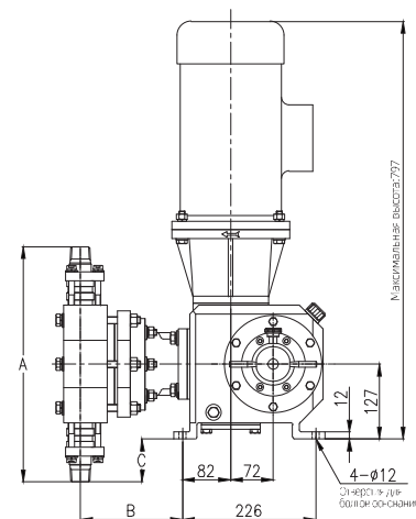
Вид сбоку
