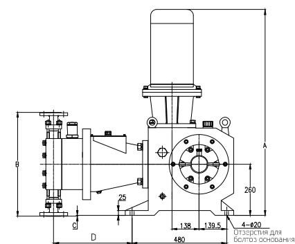
Вид сбоку
