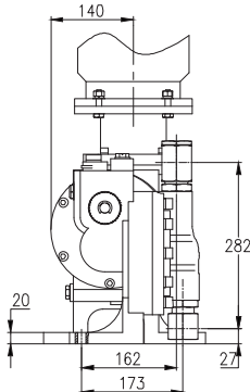
RX400-580 металлическая проточная часть вид спереди
