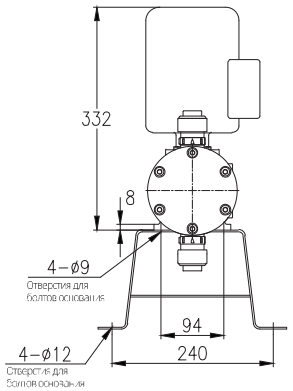
Вид спереди
