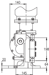
RX45-65 металлическая проточная часть вид спереди
