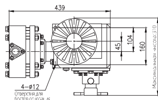
Вид спереди
