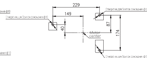
Размер отверстия для фундаментных болтов серии RB, RW
