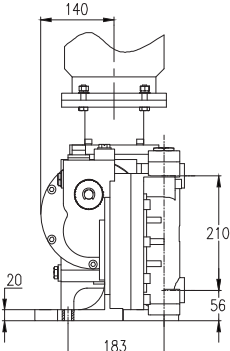
RX45-1200 металлическая проточная часть вид сбоку
