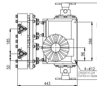
Вид спереди
